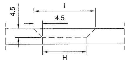
Bohrbild
