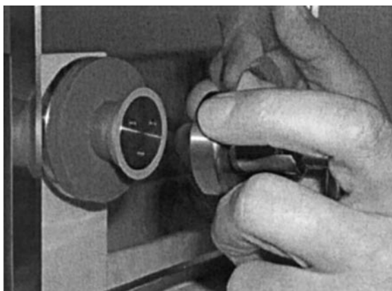
Bild 7: Senkhaltesscheibe anziehen
