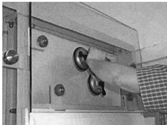
Bild 6: Glasscheibe einsetzen
